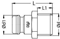
Plugs / Nippel
