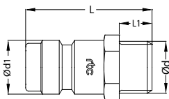
Plugs / Nippel
