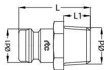
Plugs / Nippel
