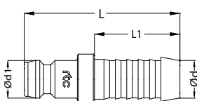
Plugs / Nippel
