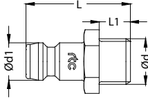
Plugs / Nippel
